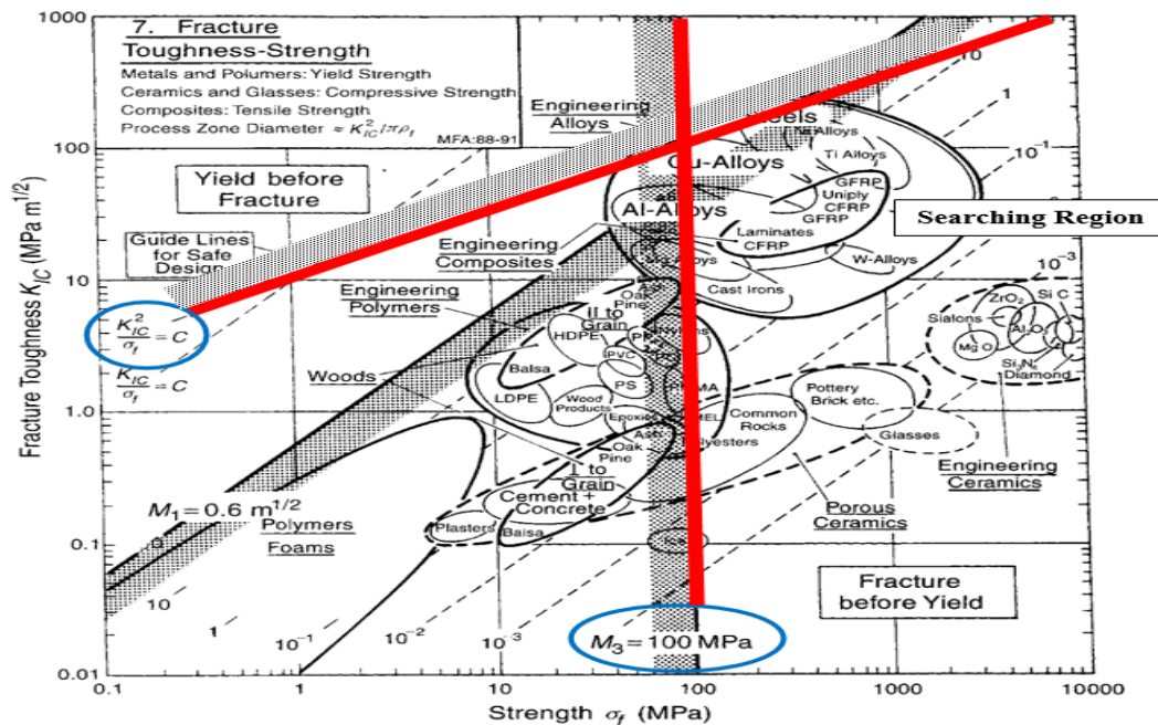
Fig 5 Chart material untuk pressure vessel [12]
