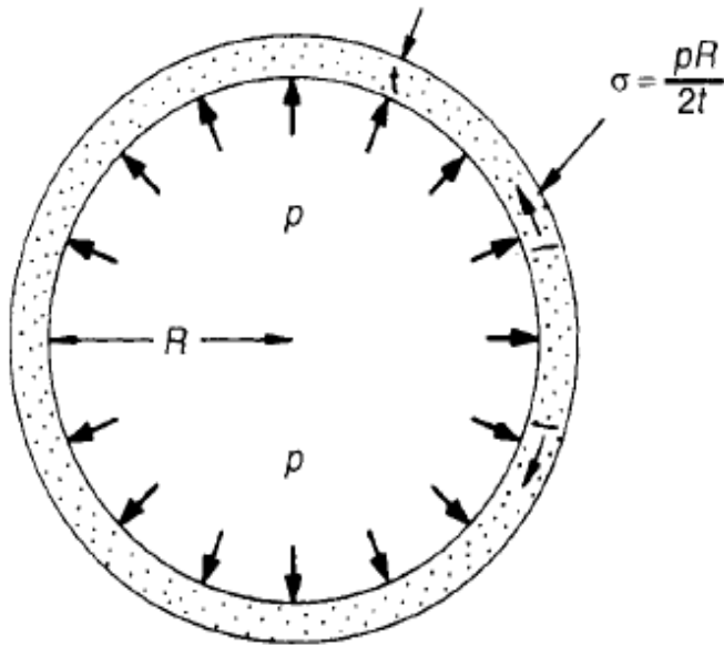
Fig 4 Skema dinding bejana CNG
