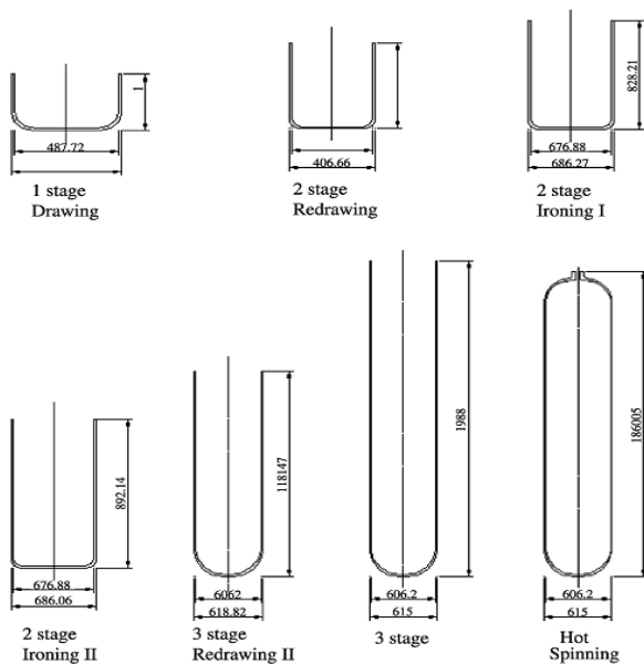
Fig 3 Ilustrasi proses produksi tabung CNG [4]
