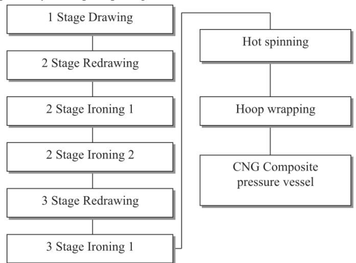
Fig 2 Alur proses produksi tabung CNG [4]
