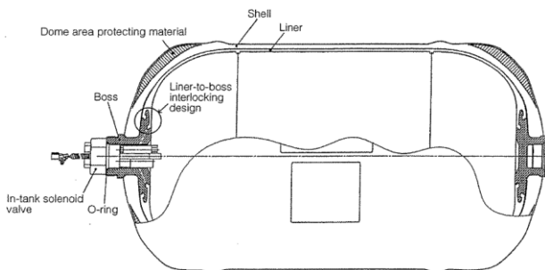
Fig 1 Skema desain tangki CNG [7]
